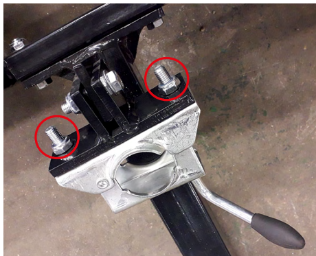
M10x35 dubbel bricka
